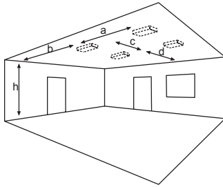
Deckenmontage
