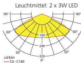
Deckenmontage
